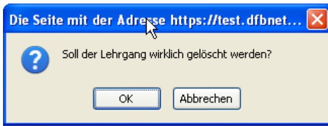
Abbildung 5 Sicherheitsabfrage
