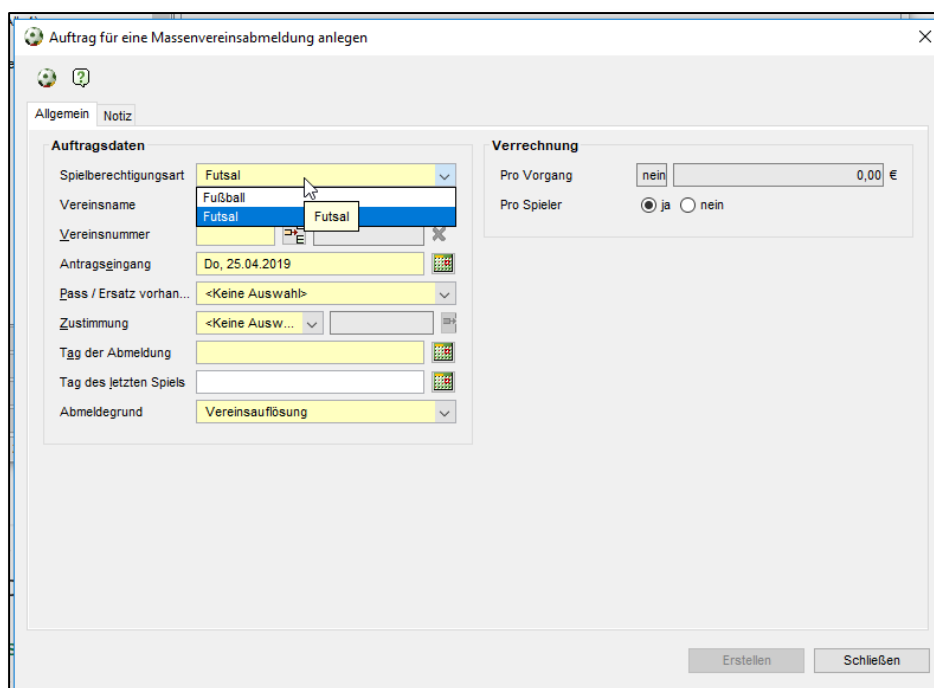
Abbildung 2: Auftrag anlegen
