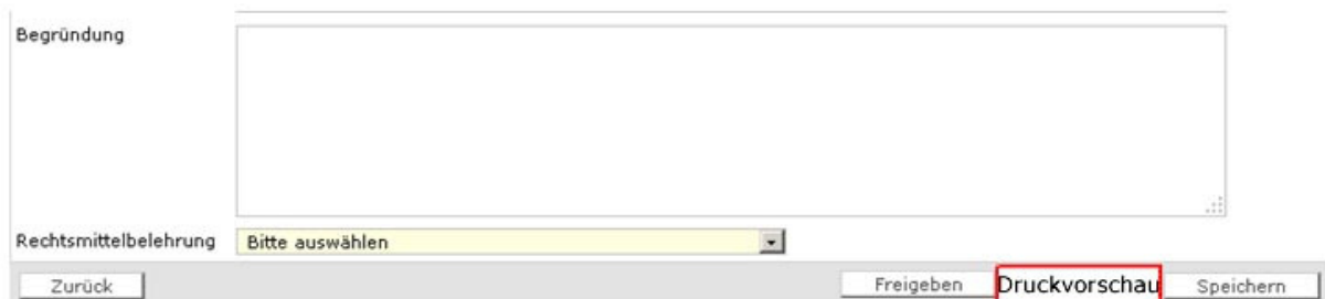
Abbildung 5 Druckvorschau
