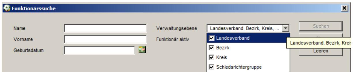
Abbildung 2: Auswahllistenfeld "Verwaltungsebene"
