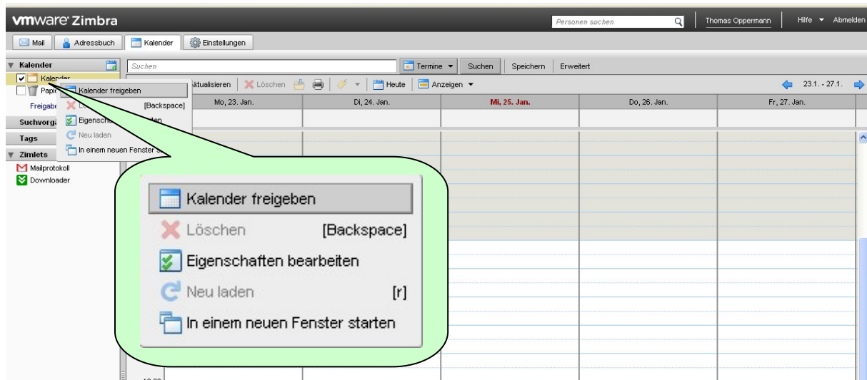
Abbildung 35: Kalender freigeben.
