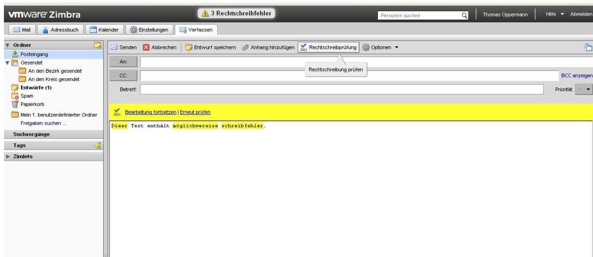
Abbildung 18: Rechtschreibprüfung starten.
