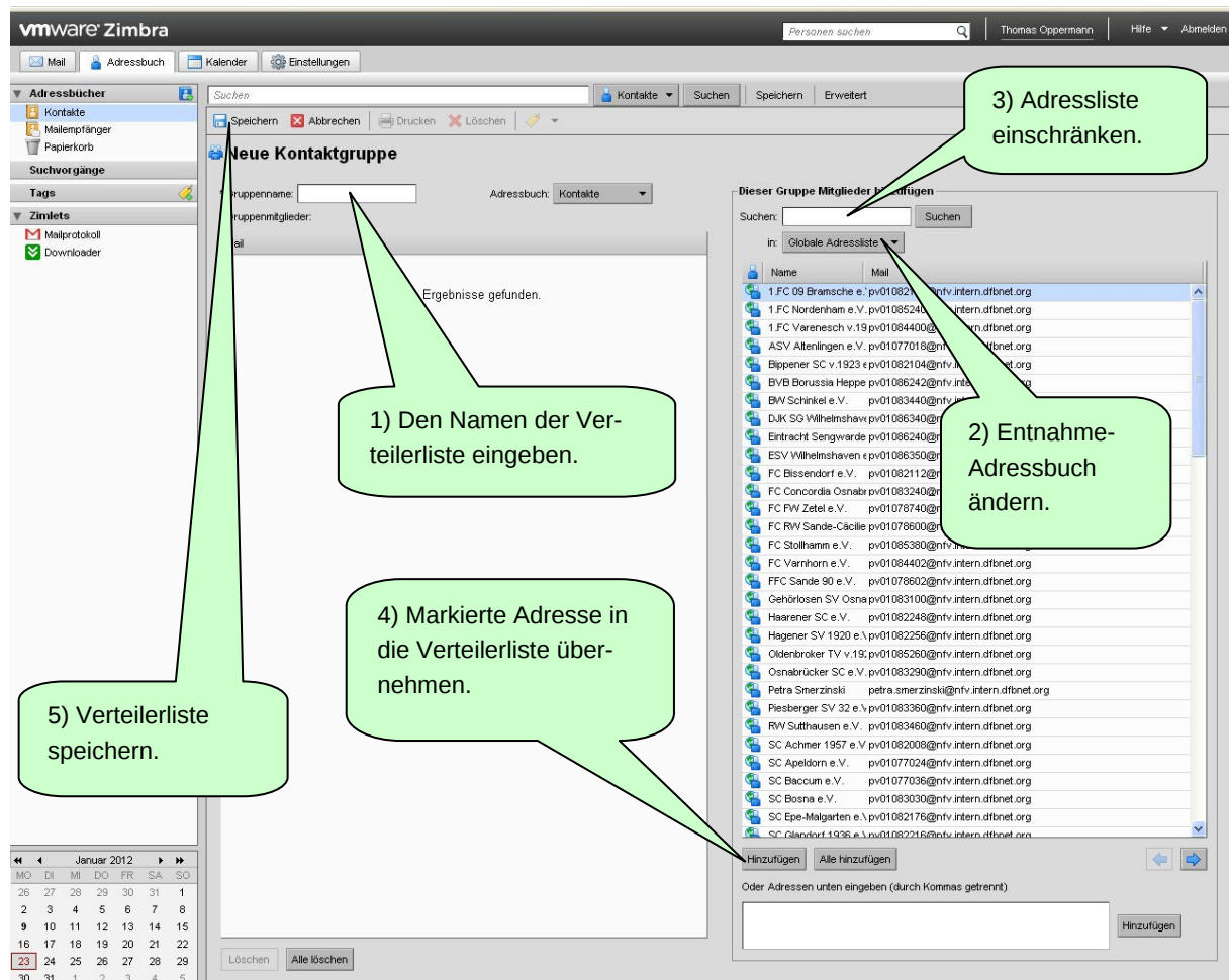
Abbildung 31: Verteilerliste erstellen.
