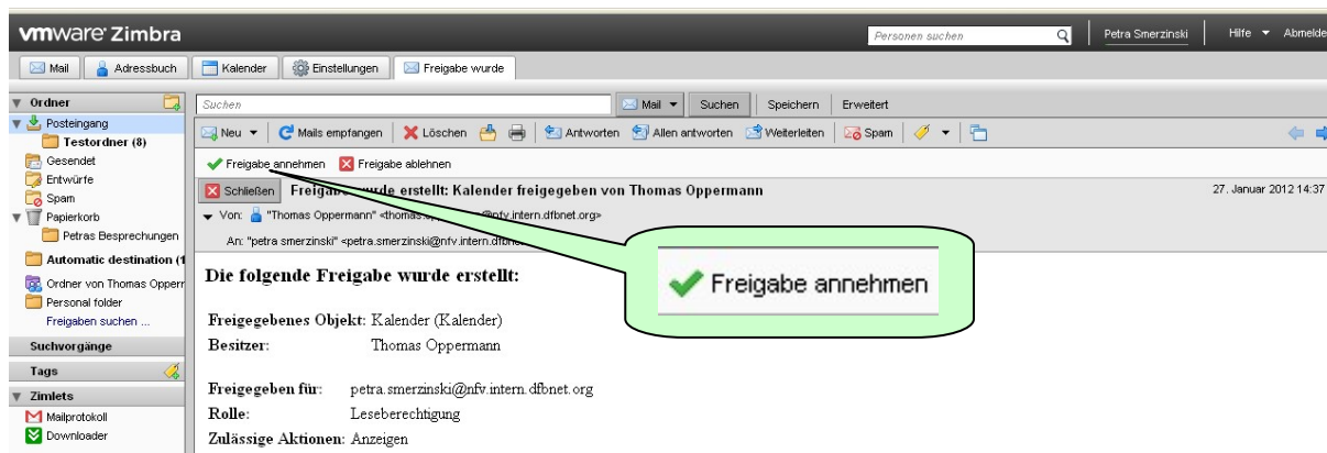
Abbildung 37: Freigabe annehmen
